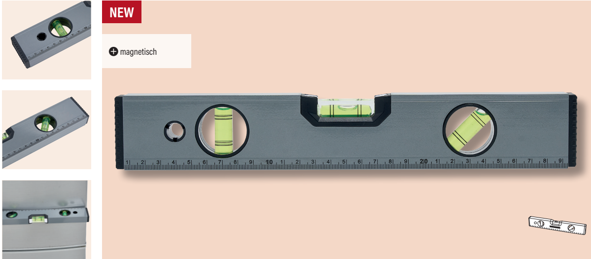
56-0380008 SODALITE Spirit level VE: 20/40 St. | Größe: 30x5x2 cm | Material: Aluminium / Acryl / Kunststoff | Veredelung: 5 cm² LY5+H2 (1) Wasserwaage: aus Aluminium, 3 separate Libellen für horizontale, vertikale und 45°-Ausrichtung, aufgedruckte Skalierung bis 30 cm, integrierter Magnet für einfache Befestigung an metallischen Oberflächen, mit gummierten Endkappen, in Box
