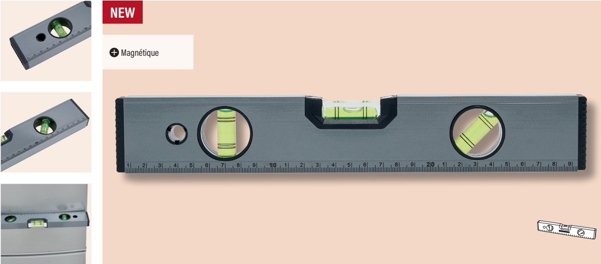
56-0380008 SODALITE Spirit level Emballage: 20/40 pcs. | Taille: 30x5x2 cm | Matériau: Aluminium / Acrylique / Plastique | Marquage: 5 cm 2 LY5+H2 (1) Niveau à bulle : en aluminium, 3 fioles séparées pour un alignement horizontal, vertical et à 45°, échelle imprimée jusqu'à 30 cm, aimant intégré pour une fixation facile sur les surfaces métalliques, embouts en caoutchouc, livré en boîte
