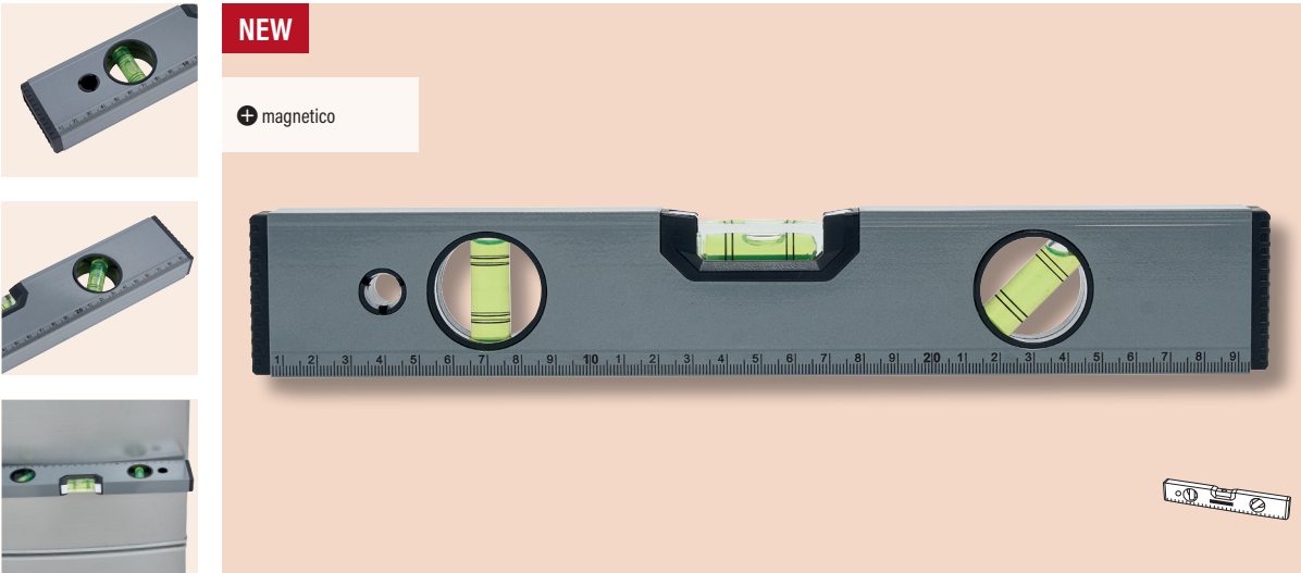
56-0380008 SODALITE Spirit level Imballo: 20/40 pz. | Dimensione: 30x5x2 cm | Materiale: alluminio / acrilico / plastica | Dimensione di stampa: 5 cm 2 LY5+H2 (1) Livella: in alluminio, 3 bolle separate per allineamenti orizzontali, verticali e a 45°, scala fino a 30 cm, magnete integrato per un facile fissaggio su superfici metalliche, con cappucci terminali in gomma, confezione in scatola
